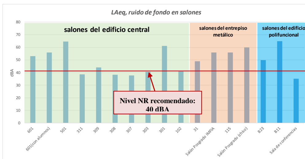
Figura 3. Niveles de ruido de fondo medidos (como L_{A,eq} ) en los salones ensayados
