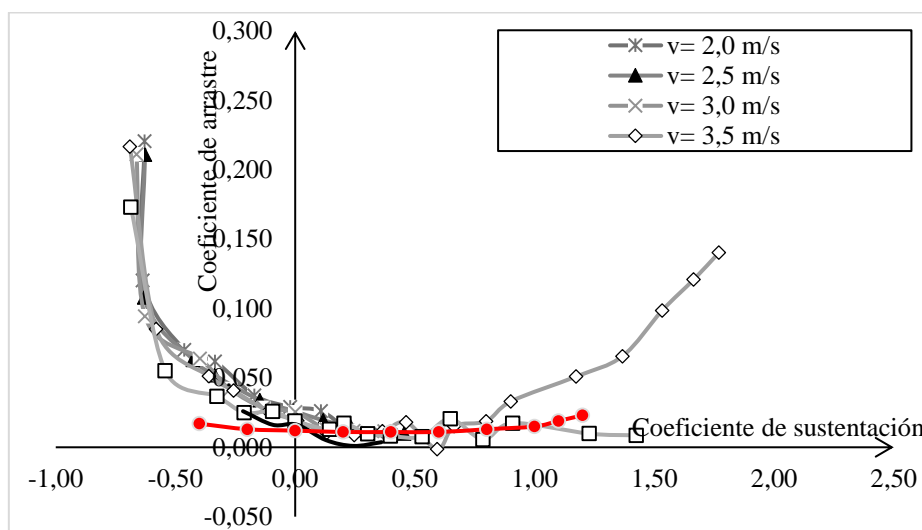
Figura 8. Relación C_L-C_D obtenida de bibliografía (curvas grises) y determinada en laboratorio (curva roja) para distintas velocidades (tomada de Abbott, 1958)
