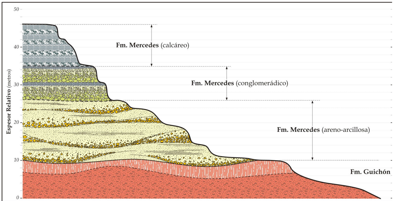
Figura 3.- Perfil esquemático de la secuencia sedimentaria
