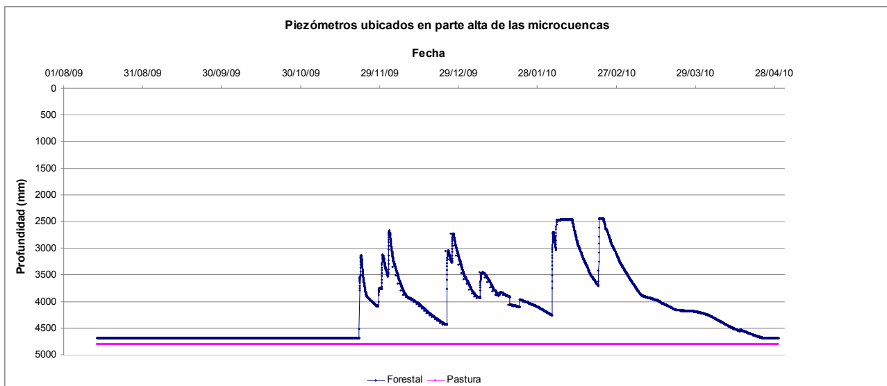
Figura 8.- Recuperación de niveles piezométricos, ubicación alta
