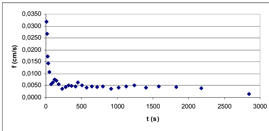
Figura 5.- Ensayo de infiltración en el piezómetro, ubicado en la posición media, en la microcuenca La Cantera (pasturas naturales)
