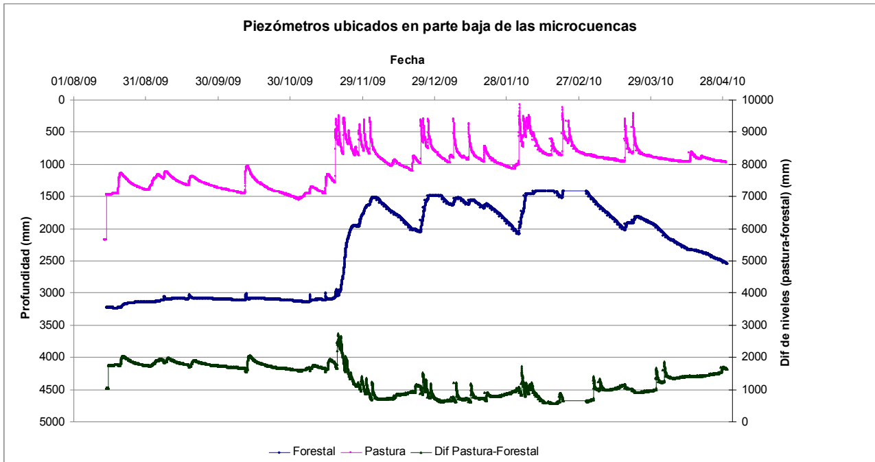
Figura 6.- Recuperación de niveles piezométricos, ubicación baja
