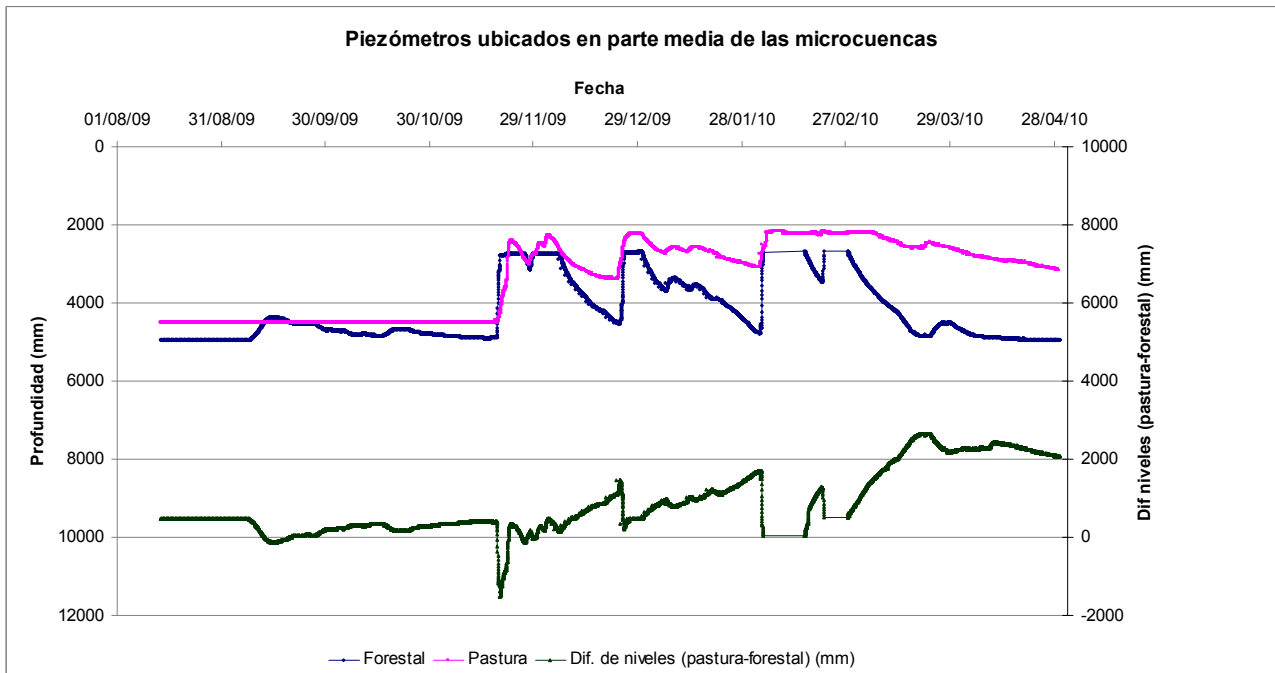
Figura 7.- Recuperación de niveles piezométricos, ubicación media
