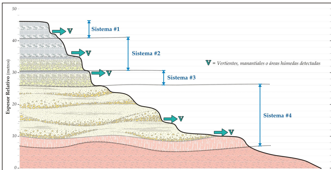
Figura 4.- Sistema de acuíferos colgados
