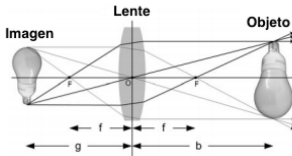
Figura 2.4: Lente. La figura muestra cómo los rayos de un objeto (una lamparita) se enfocan a través del lente. La bombita real se encuentra a la izquierda y la imagen formada a la derecha [20, Figura 2.6, Página 12].
