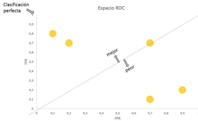
Figura 5.2: Curva ROC
