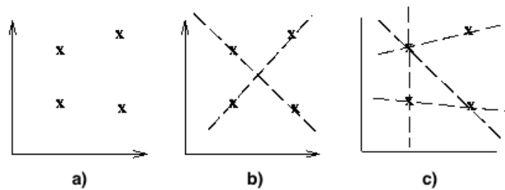
Figura 2.24: a) Coordenadas de puntos , b) y c) posibles rectas formadas a partir de los puntos .
