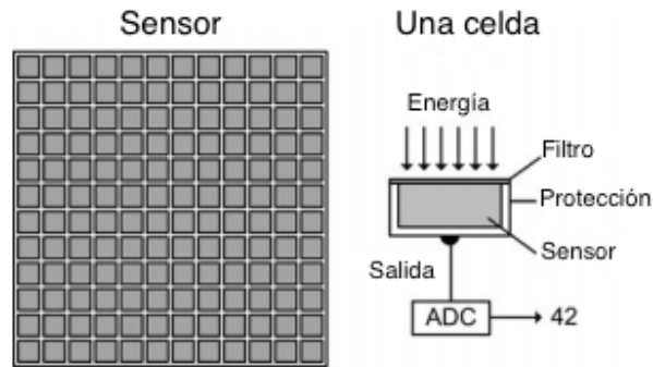
Figura 2.5: Sensor. El sensor consiste de un arreglo de celdas interconectadas. Cada celda consiste de una protección que soporta el filtro, un sensor y una salida. El filtro controla qué tipo de energía es permitida entrar al sensor. El sensor mide la cantidad de energía como voltaje, que luego es convertido a un número digital a través de un conversor análogo-digital (ADC) [20, Figura 2.13, Página 17].
