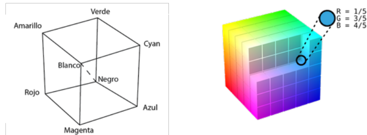
Figura 2.9: Cubo RGB.
