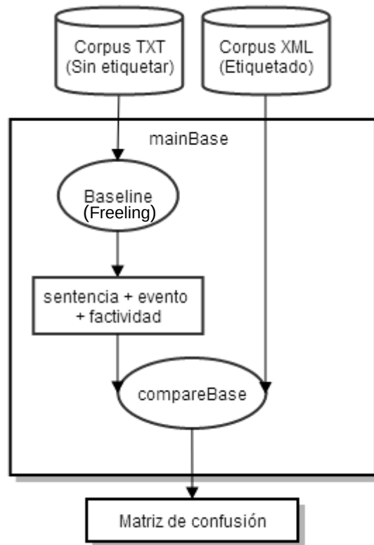
Figura 20 – Diagrama de la línea base
