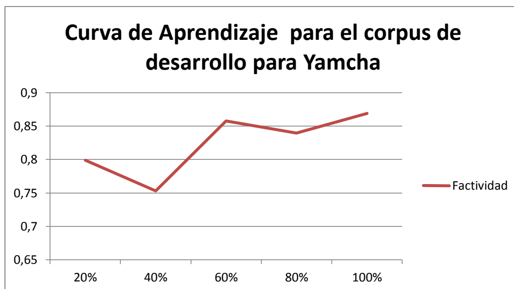
Gráfico 2 - Curva de aprendizaje del corpus de desarrollo para Yamcha
