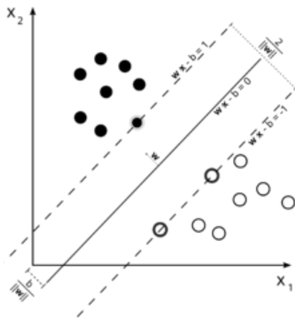
Figura 14 - Ejemplo de SVM
