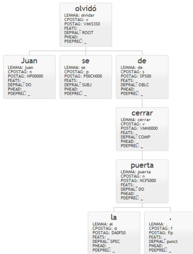
Figura 13 - Árbol de dependencias de (6.18)
