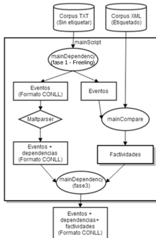
Figura 21 – Diagrama de la construcción de los archivos en formato CONLL
