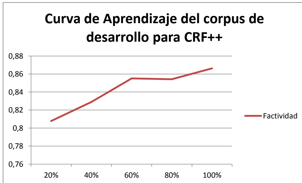
Gráfico 1 - Curva de aprendizaje del corpus de desarrollo para CRF++
