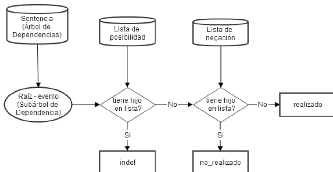
Figura 1 - Diagrama de la línea base inicial
