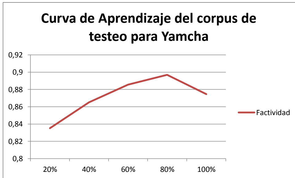
Gráfico 4 - Curva de aprendizaje del corpus de testeo para Yamcha
