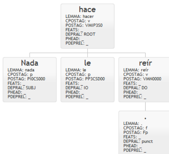
Figura 9 - Árbol de dependencias de (6.11)
