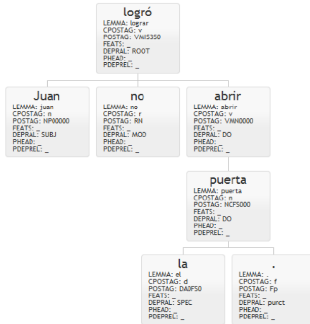
Figura 12 - Árbol de dependencias de (6.17)
