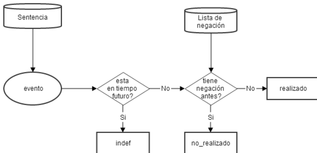
Figura 2 - Diagrama de la línea base final
