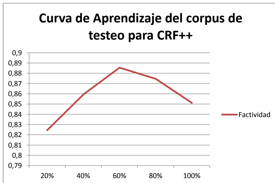
Gráfico 3- Curva de aprendizaje del corpus de testeo para CRF++
