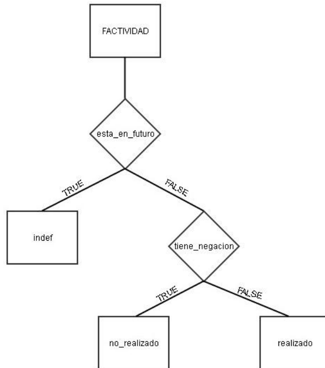
Figura 15 - Ejemplo de un árbol de decisión
