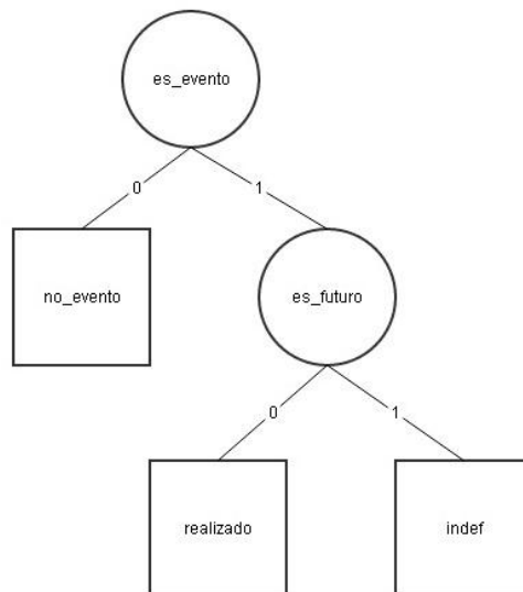
Figura 23 - Árbol de decisión formado por Weka
