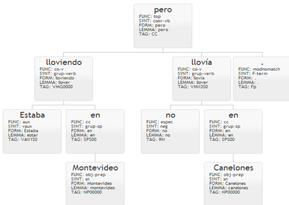
Figura 16 - Árbol de dependencias del ejemplo (7.1)
