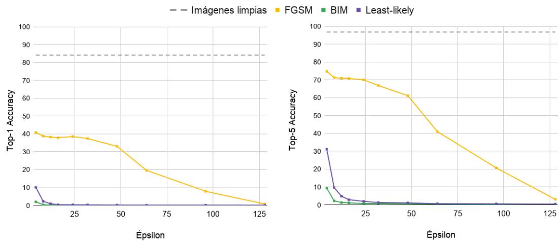
Figura 5.2: Accuracy obtenida por los métodos FGSM, BIM e Iterative least-likely en una red Inception-v3 para distintos valores de \epsilon .
