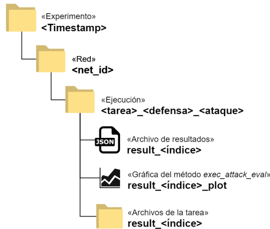
Figura 4.2: Estructura de directorios utilizada para almacenar los resultados de los experimentos.
