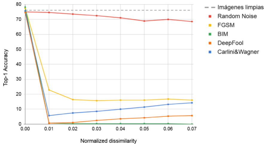
Figura 5.5: Accuracy de la red ResNet-50 sobre ejemplos adversarios de distintos ataques para múltiples valores de normalized dissimilarity .
