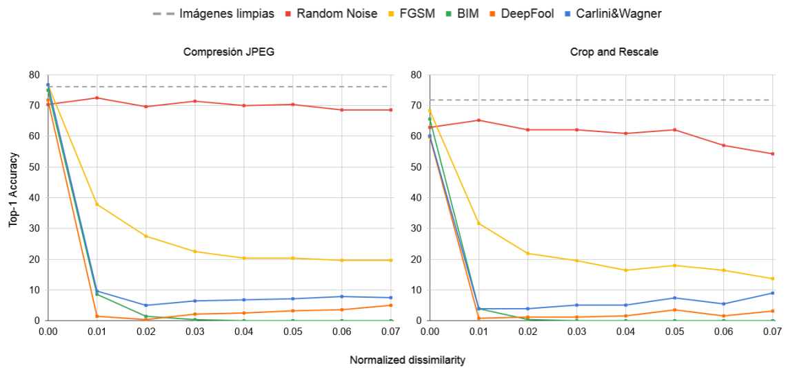
Figura 5.7: Accuracy obtenida para múltiples valores de normalized dissimilarity sobre imágenes generadas por los distintos ataques implementados en una red ResNet-50, utilizando los mecanismos de defensa Compresión JPEG (izquierda) y Crop and Rescale (derecha) en modalidad white-box , aplicando BPDA y EOT respectivamente.
