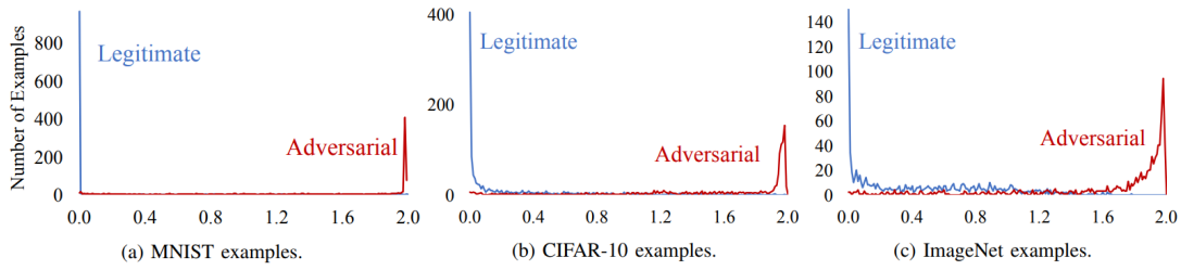
Figura 3.7: Diferencia (en norma L_1 ) entre la predicción realizada sobre la imagen original y la predicción realizada sobre la imagen después de aplicar las transformaciones squeeze definidas por la defensa. En azul se indica esta diferencia para las imágenes legítimas mientras que en rojo la diferencia para imágenes con perturbaciones adversarias, destacando que se pueden diferenciar ambos casos claramente.
