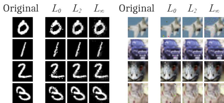
Figura 3.1: Ejemplos adversarios generados por el ataque Carlini&Wagner [15] sobre los datasets MNIST y CIFAR-10. En la primera columna de cada dataset se presentan imágenes limpias, las siguientes tres presentan ejemplos adversarios optimizados para las normas L_0 , L_2 y L_\infty respectivamente.
