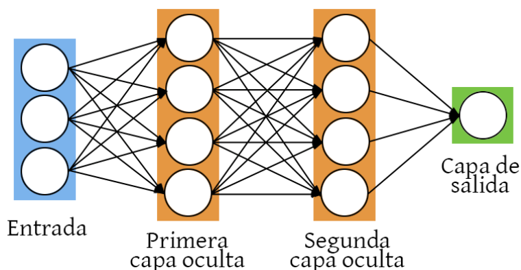
Figura 2.1: Diagrama de una red neuronal prealimentada de dos capas ocultas.
