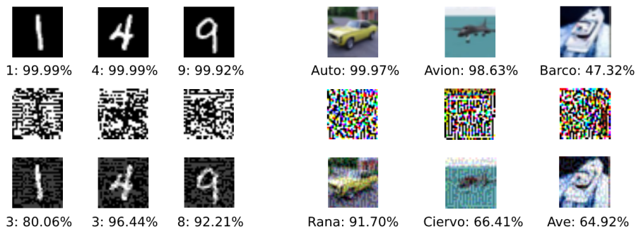
Figura 5.1: Ejemplos de perturbaciones generadas por el FGSM sobre los datasets MNIST y CIFAR-10 con valores de \epsilon de 0,25 y 0,1 respectivamente (rango de 0 a 1). En cada caso se muestra la clase y probabilidad asignada por la red.
