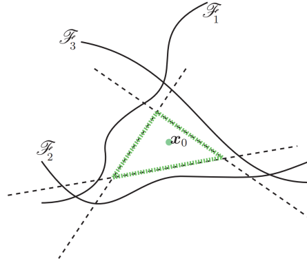
Figura 3.3: Representación de la región P considerada por el método DeepFool y su aproximación mediante el poliedro \tilde{P} alrededor de un punto x_0 .
