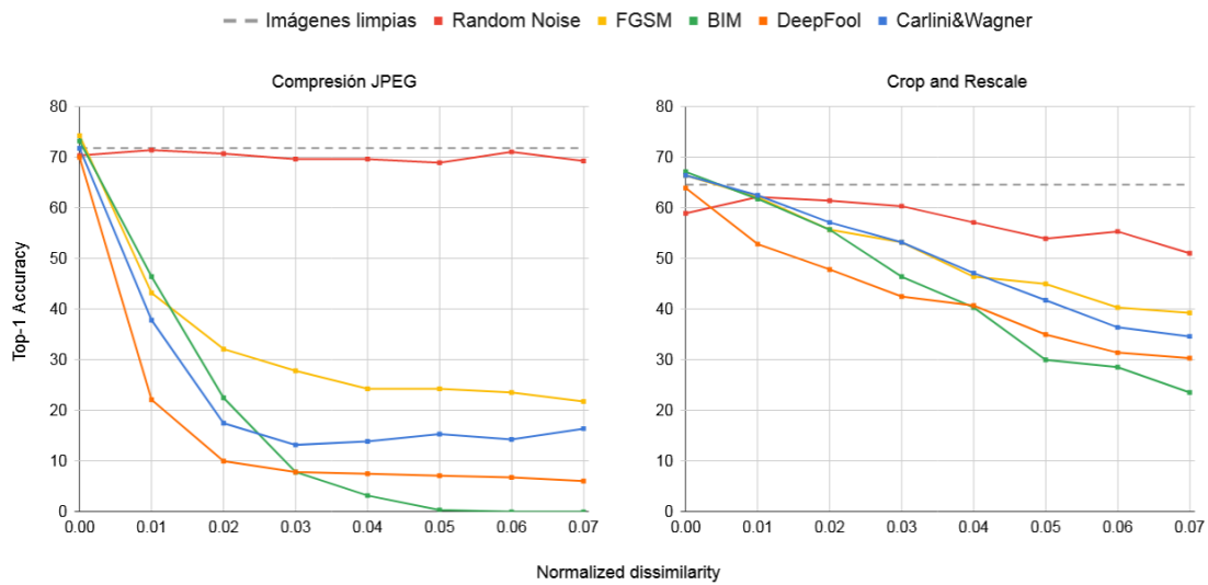
Figura 5.6: Accuracy obtenida para múltiples valores de normalized dissimilarity sobre imágenes generadas por los distintos ataques implementados en una red ResNet-50, utilizando los mecanismos de defensa Compresión JPEG (izquierda) y Crop and Rescale (derecha).
