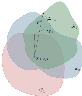
Figura 3.4: Representación del algoritmo Universal Adversarial Perturbations . En esta se representa el vector de perturbación r^* generado a partir de tres imágenes x_1 , x_2 y x_3 las cuales se muestran superpuestas por simplicidad.
