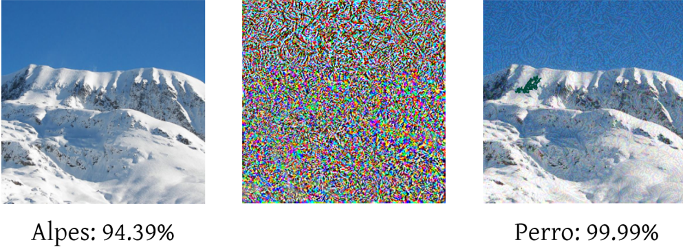
Figura 3.2: Ejemplo adversario generado con el método MI-FGSM. En esta se puede observar la imagen limpia seguida de la perturbación adversaria y el ejemplo resultante, indicando en ambos casos la clase asignada por la red.
