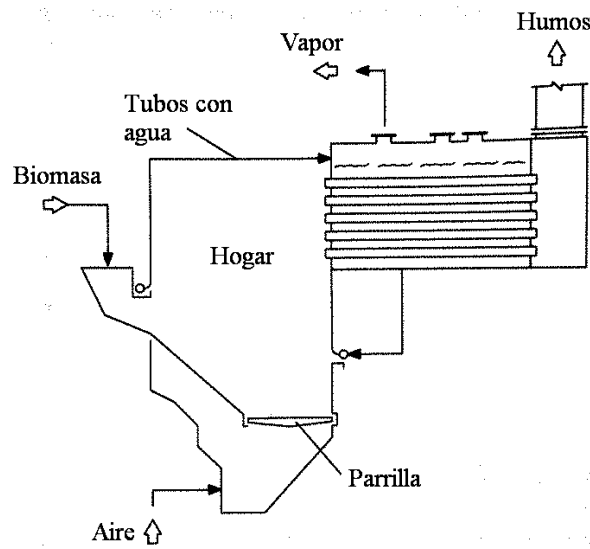
Figura A.1: Generador de vapor humotubular de hogar exterior para quema de biomasa. [22]
