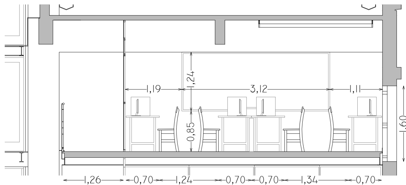
CORTE A-A
