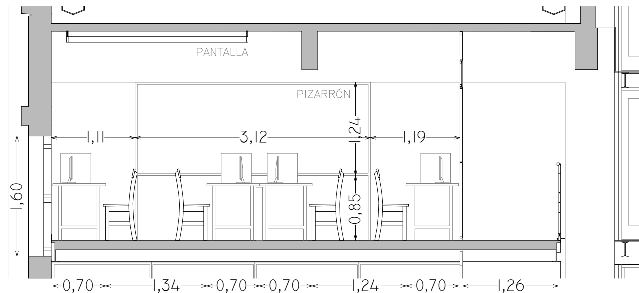
CORTE A-A
