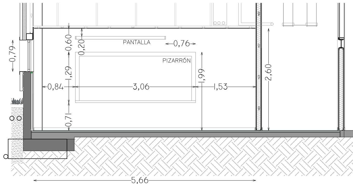
CORTE A-A
