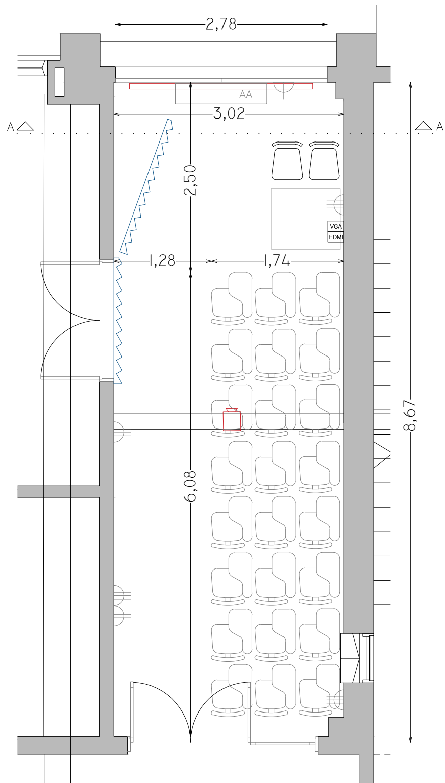
PLANTA
