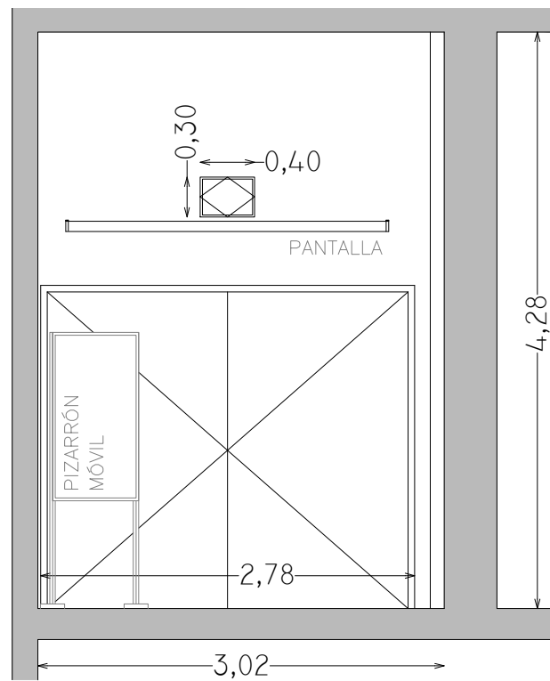
CORTE A-A
