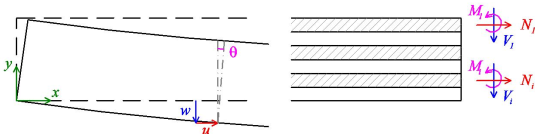
Figura 4.2: Desplazamientos y solicitaciones incógnitas en el problema de flexión.
