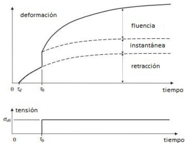
Figura 2.7: Deformaciones instantáneas y diferidas.
