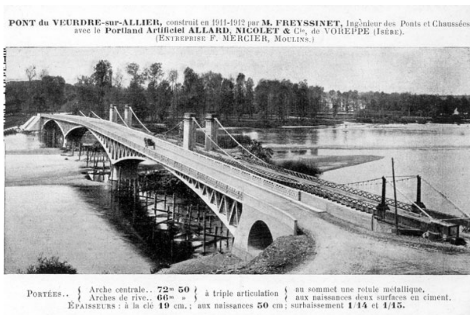
Figura 1.1: Puente Le Veudre.
