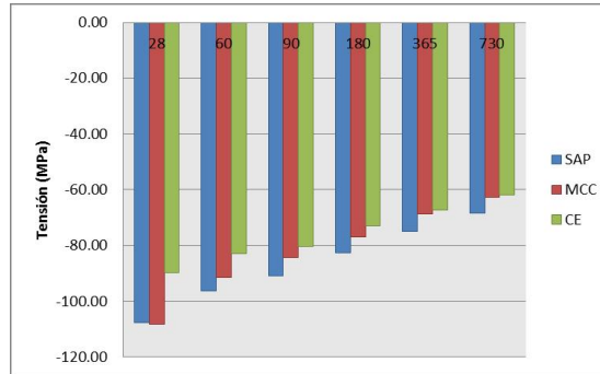
Figura 6.22: Comparación de la tensión en la fibra superior del hormigón obtenida mediante el SAP, MCC y CE.
