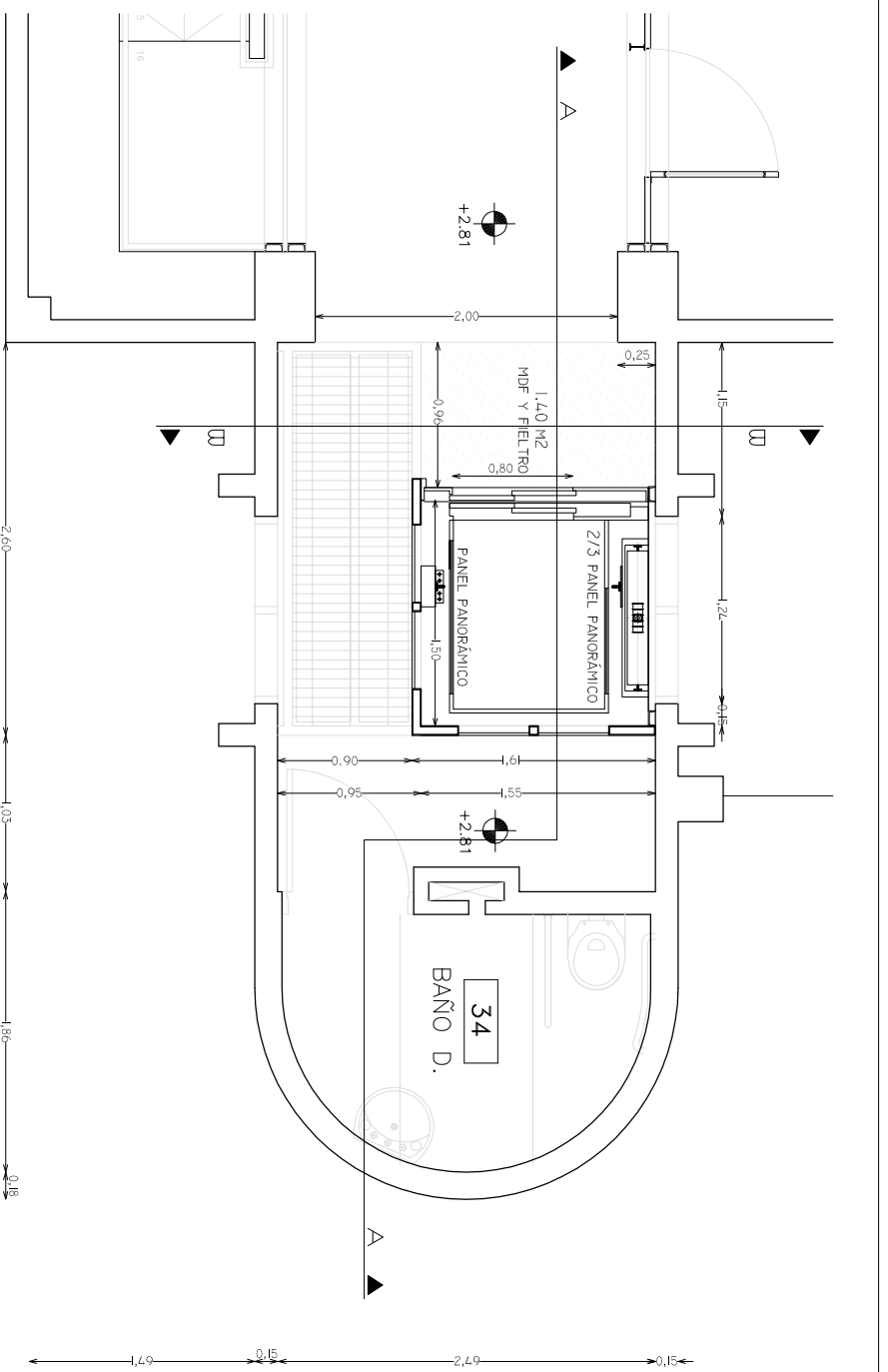
PARADA 3 NIVEL +2.81 ESC.: 1/50
