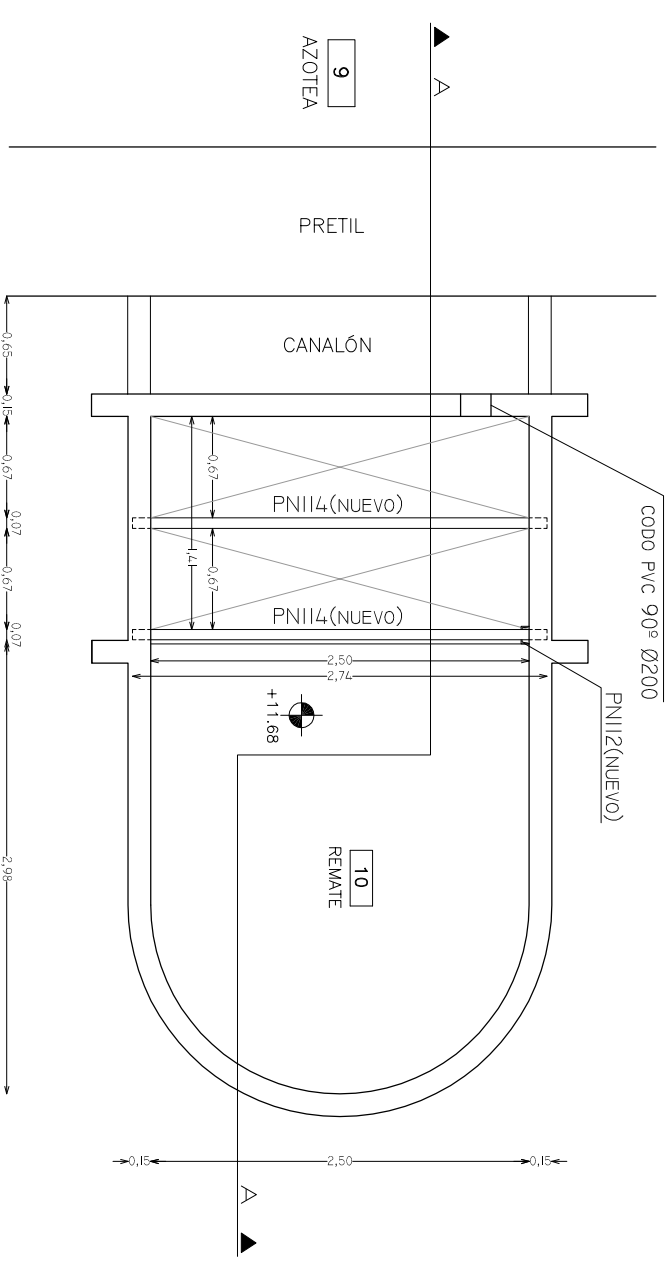
PLANTA ESTRUCTURA NIVEL 3 - 4 - 5 ESC.: 1/50
