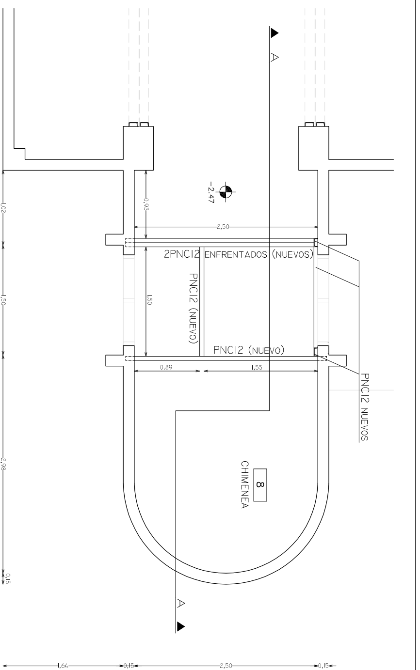
PLANTA ESTRUCTURA NIVEL 1 ESC.: 1/50
