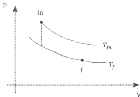
Camino de cálculo para la entropía del gas ideal en el ejercicio 3
