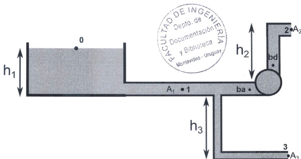
Figura 1: Puntos de referencia para aplicar Bernoulli en el ejercicio 2
